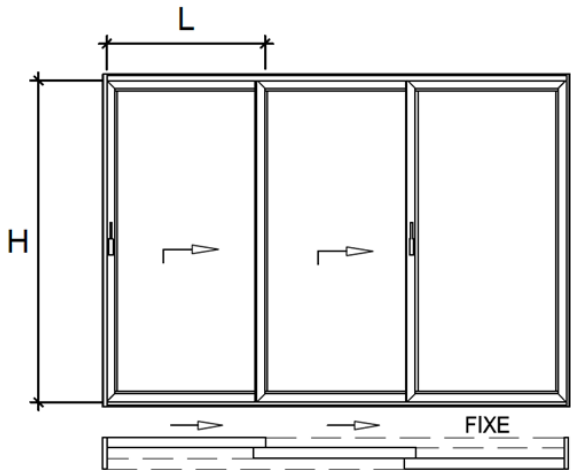
2 Panneaux coulissants + 1 Panneau fixe ou 3 Panneaux coulissants
