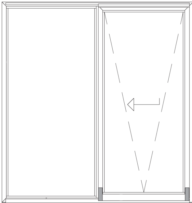
Porte-fenêtre oscillo-coulissante, périmètre régulier 2 3/8" avec extension, volet robuste
